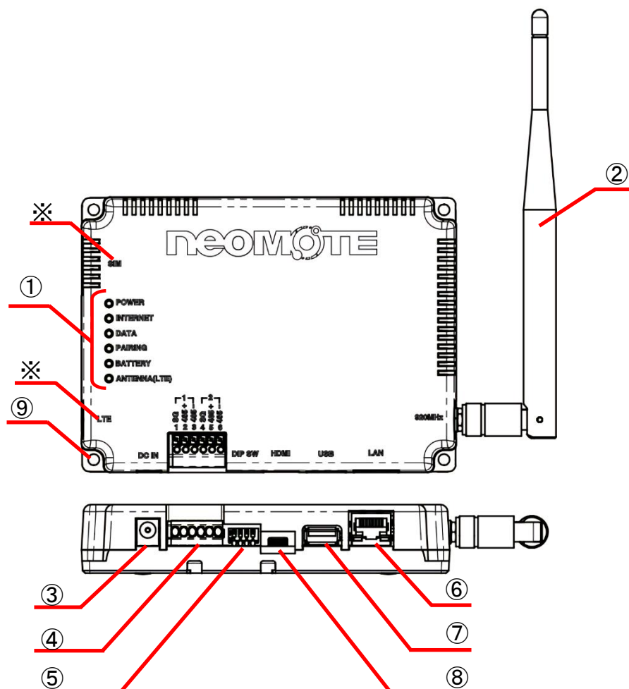
図2 各部名称
