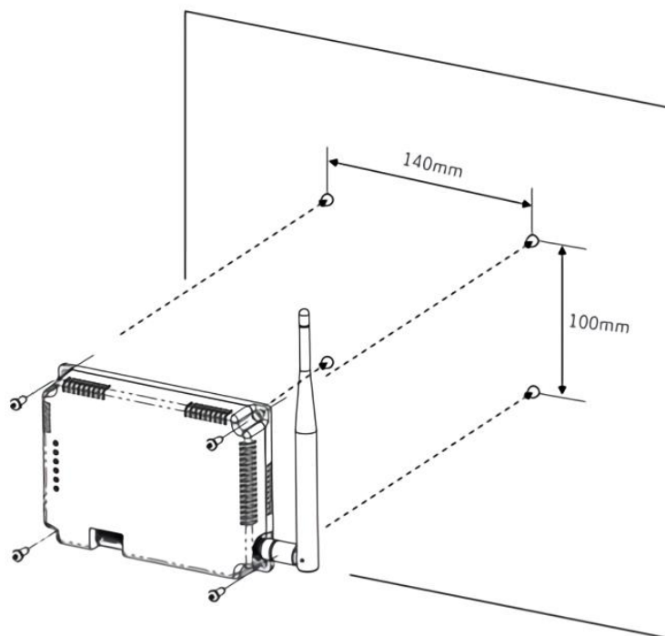
図 49 ゲートウェイ取り付け方法 1
