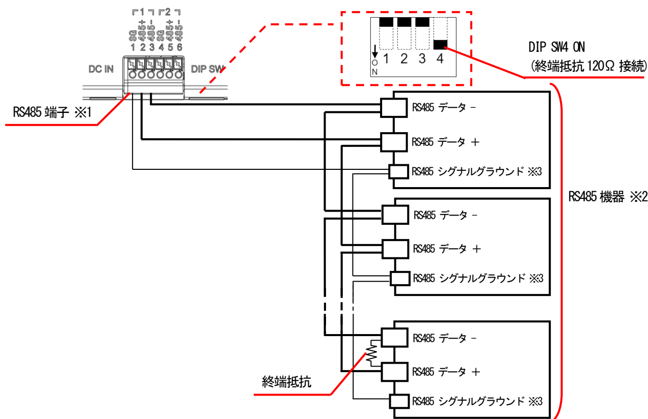
図 51 RS485 配線
