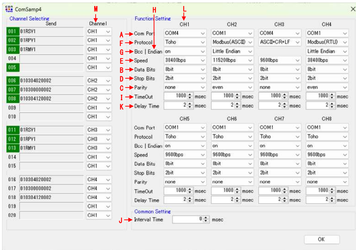
ゲートウェイモード
