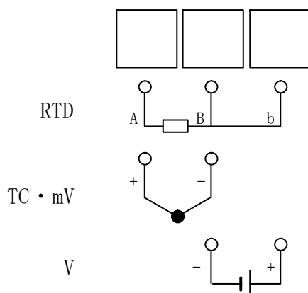
CH共通 入力種類別配線方法
