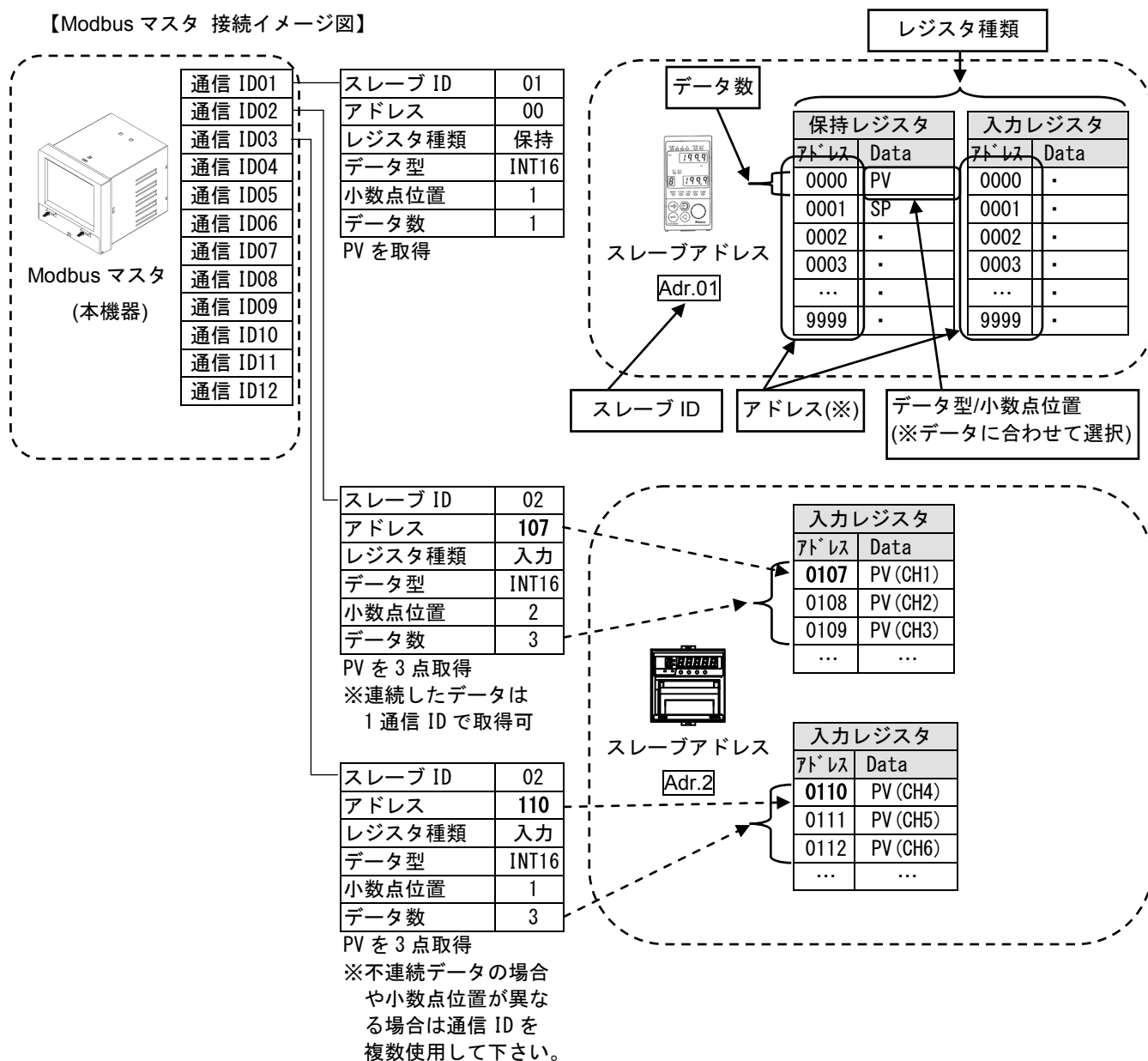
【Modbus マスタ 演算チャネル割付イメージ】
